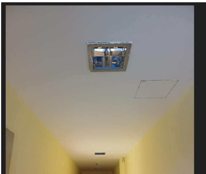
Obrázek 3 - strop chodba
